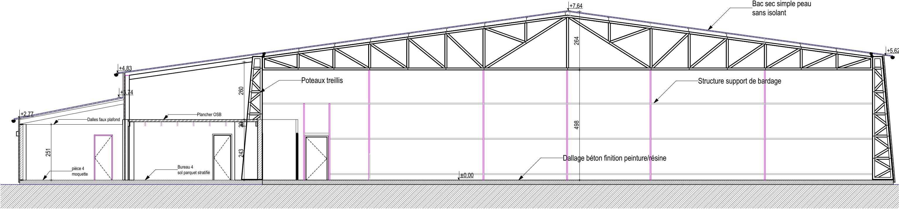
Coupe AA
