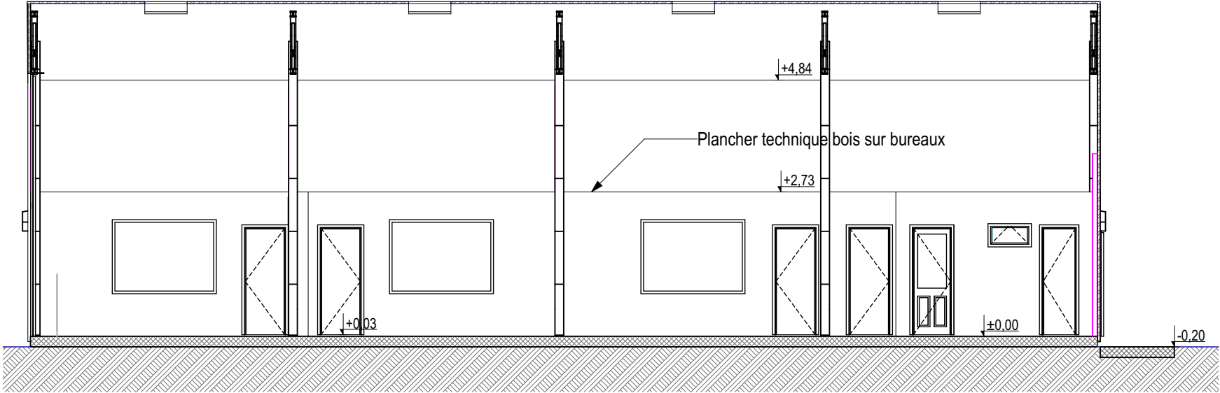
Coupe BB
